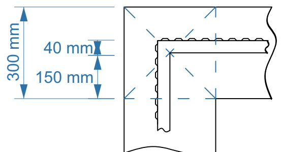
A fémgarázs elhelyezése a betongyűrű alapon
