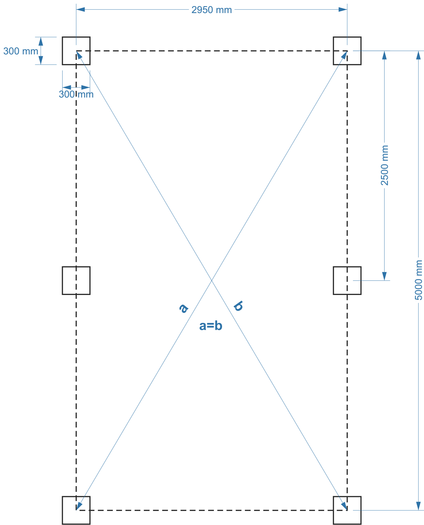
Betonkocka alap
